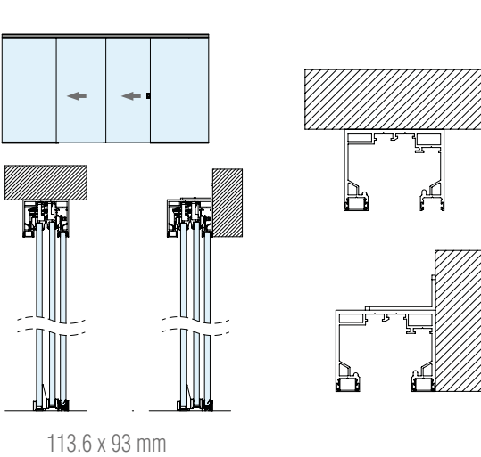
TELESCOPICO CON VETRO FISSO Telescopic with Sidelight
