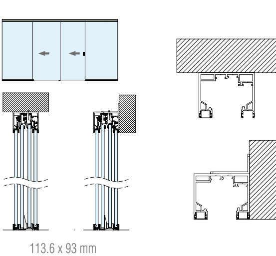
TELESCOPICO CON DOPPIO VETRO FISSO Sliding with double Sidelight
